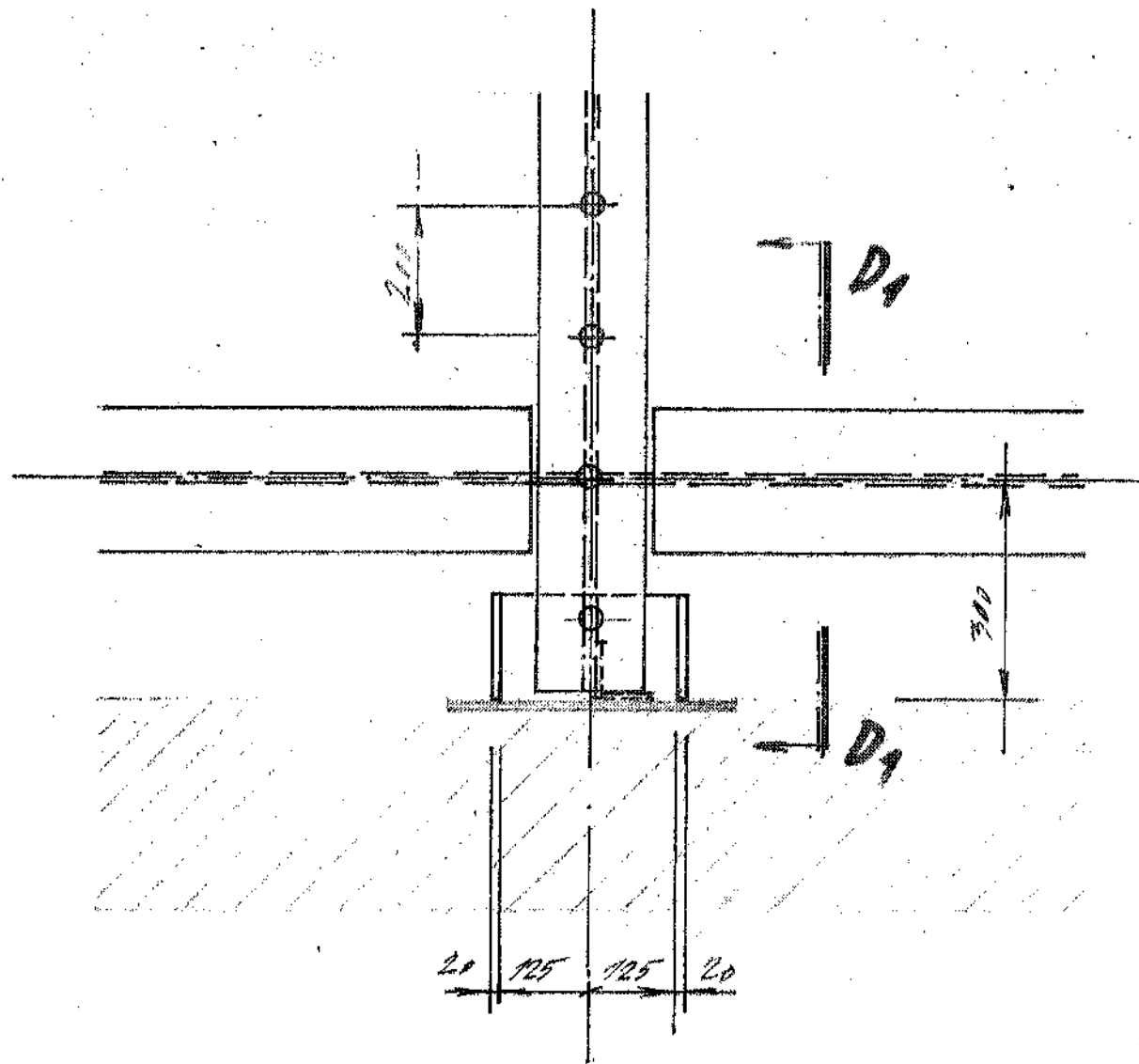
ŘEZ E 1 -E 1 Section
