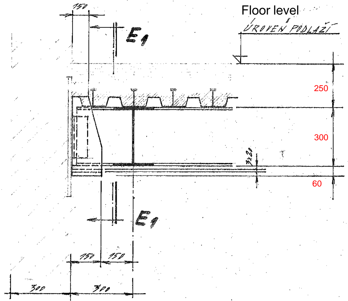
ŘEZ D 1 -D 1 Section
